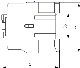
Рисунок 2 – Габаритные и установочные размеры КМИе-1091(0/1), КМИе-1121(0/1), КМИе-1181(0/1), КМИе-2251(0/1)
