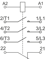
Рисунок 1 – Электрические схемы контакторов
