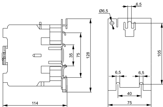
Рисунок 4 – Габаритные и установочные размеры КМИе-34012, КМИе-35012, КМИе-46512
