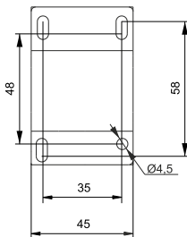
Рисунок 2 – Габаритные и установочные размеры КМИе-1091(0/1), КМИе-1121(0/1), КМИе-1181(0/1), КМИе-2251(0/1)
