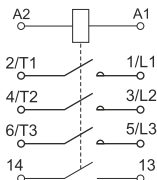
Рисунок 1 – Электрические схемы контакторов
