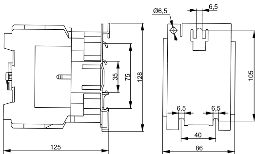
Рисунок 5 – Габаритные и установочные размеры КМИе-48012, КМИе-49512
