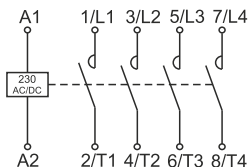
Рисунок 2 – Схемы электрические контакторов
