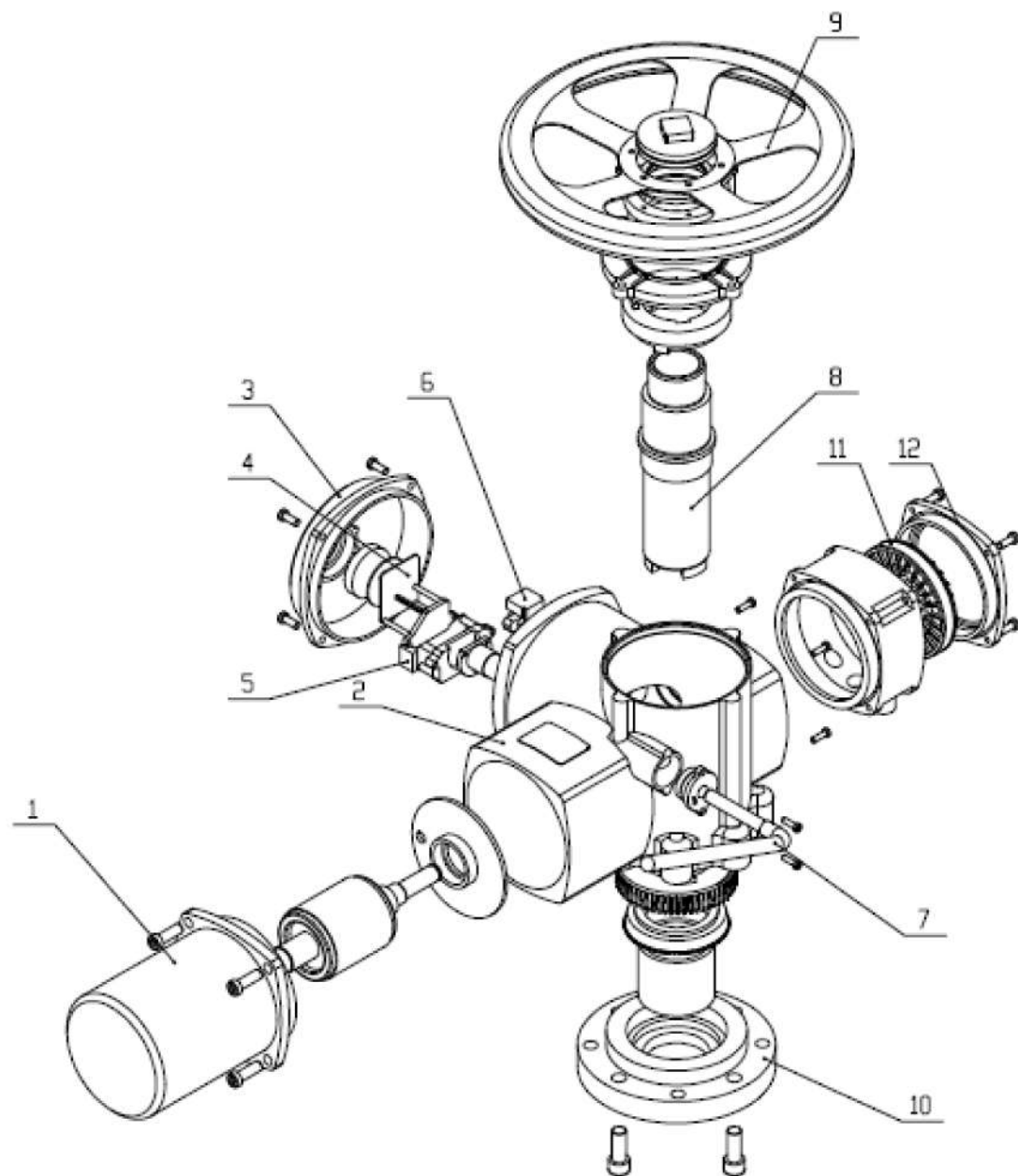
Рис.1 Устройство электропривода.
