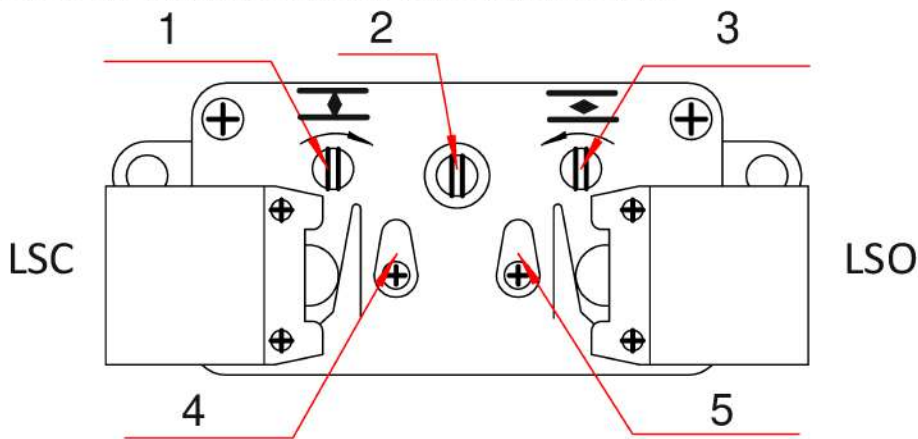
Рис. 3 Схема устройства ограничения хода выходного вала.
